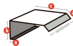
ESQUINERO 2P
